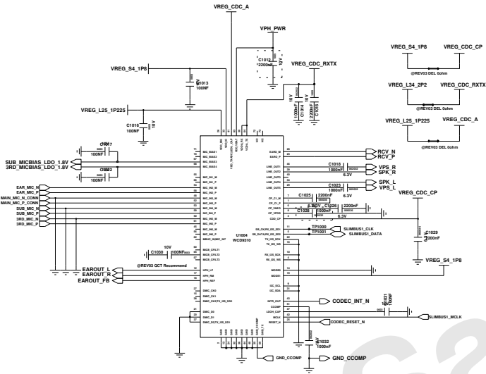
AUDIO CODEC
